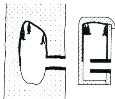
Vergleich der Querschnitte einer natürlichen Baumhöhle und des Rundkastens
